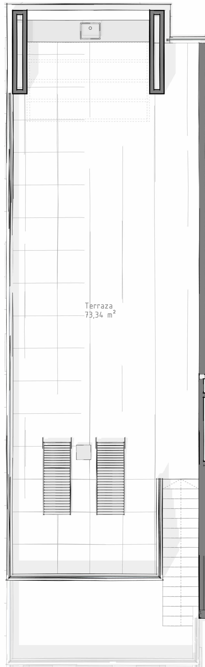
Bloque 2. Viv A. Solarium
