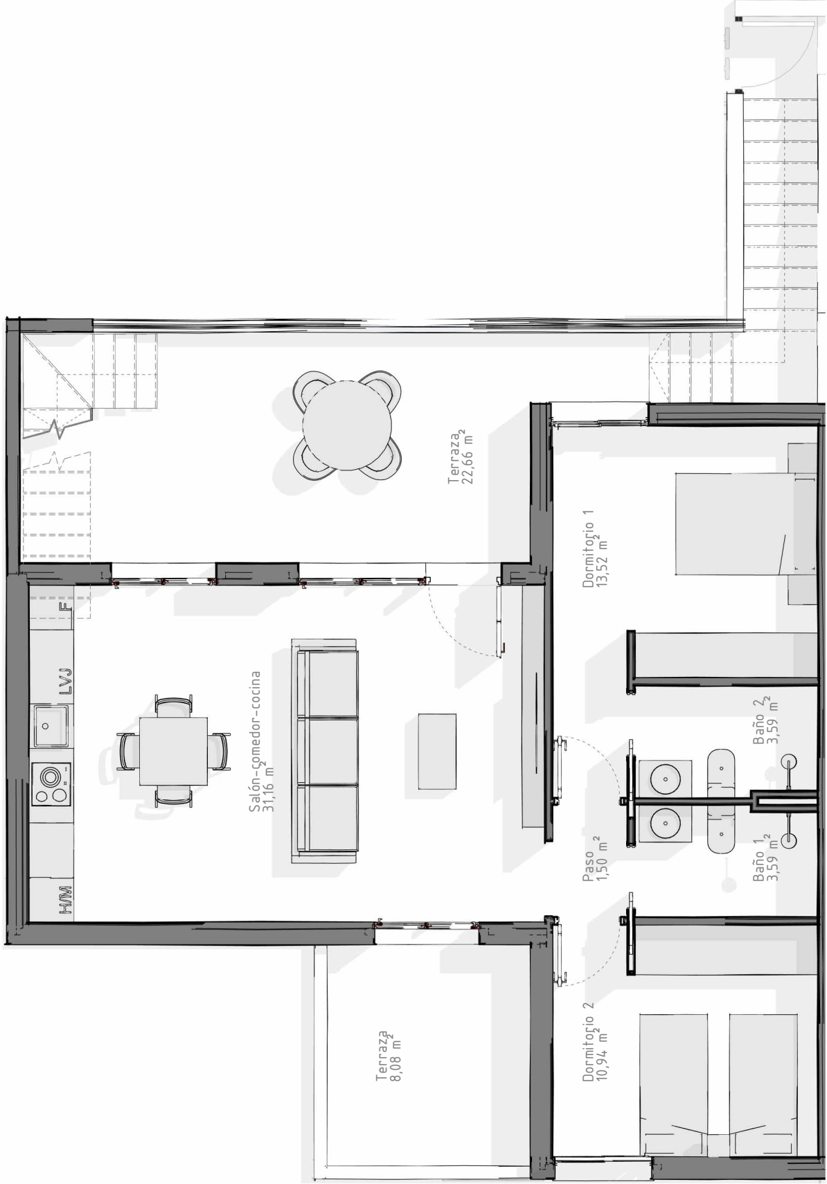
Planta alta
